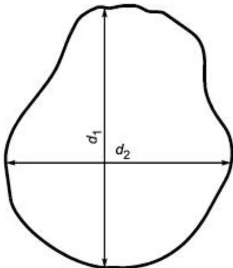
Рисунок 7 - Измерение расплыва бетонной смеси
