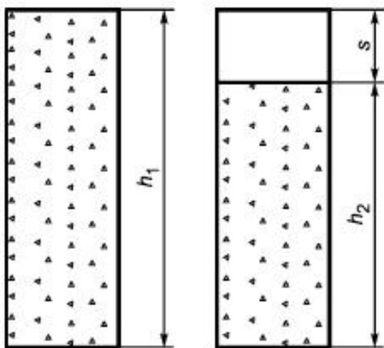
Рисунок 8 - Форма для определения степени уплотняемости бетонной смеси
